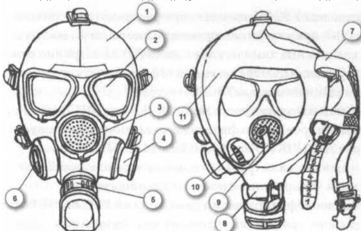
Рис. 26. Устройство гражданского противогаза ГП-9. 1 — корпус; 2 — очковый узел; 3 — переговорное устройство; 4 — узел вдоха; 5 — узел выдоха; 6 — заглушка; 7 — наголовник; 8 — клапанный узел приспособления для приема воды; 9 — мундштук; 10 — обтекатель; 11 — «независимый» обтюратор Источник: Сайт ОАО «ЭХМЗ имени Н.Д. Зелинского» ( www.ehmz.ru )
